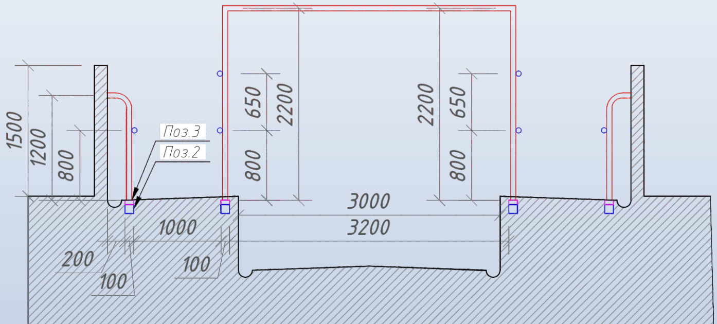
РАЗРЕЗ ДОИЛЬНОГО ЗАЛА
